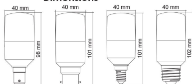
Dimensions
