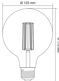
LG125 E27
